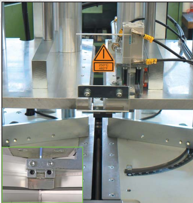
With optional gasket moulder / Avec option - presseur de joint.
